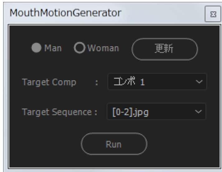
図 1 GUI
