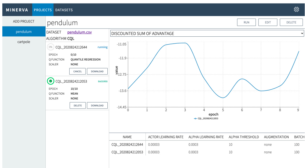
図3. MINERVAのUI
