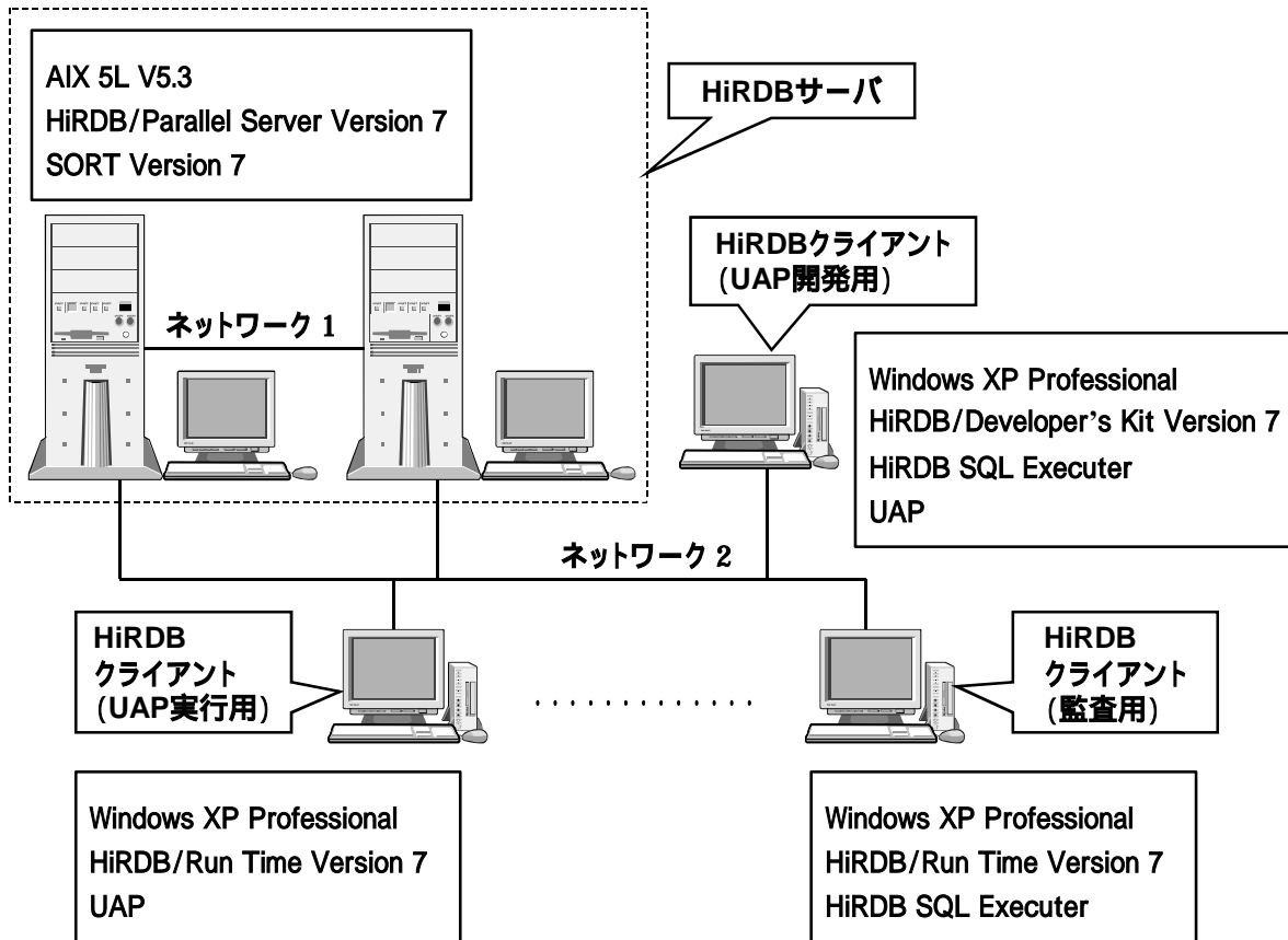
図 2-1 : クライアント - サーバ(C/S)型のシステム構成
