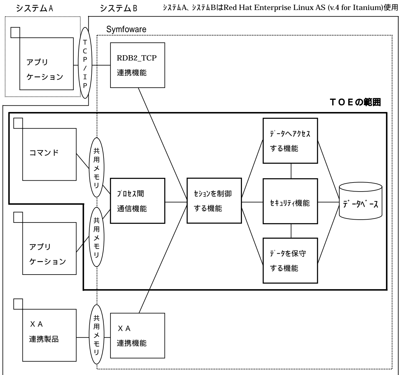
図 1-2 機能構成
