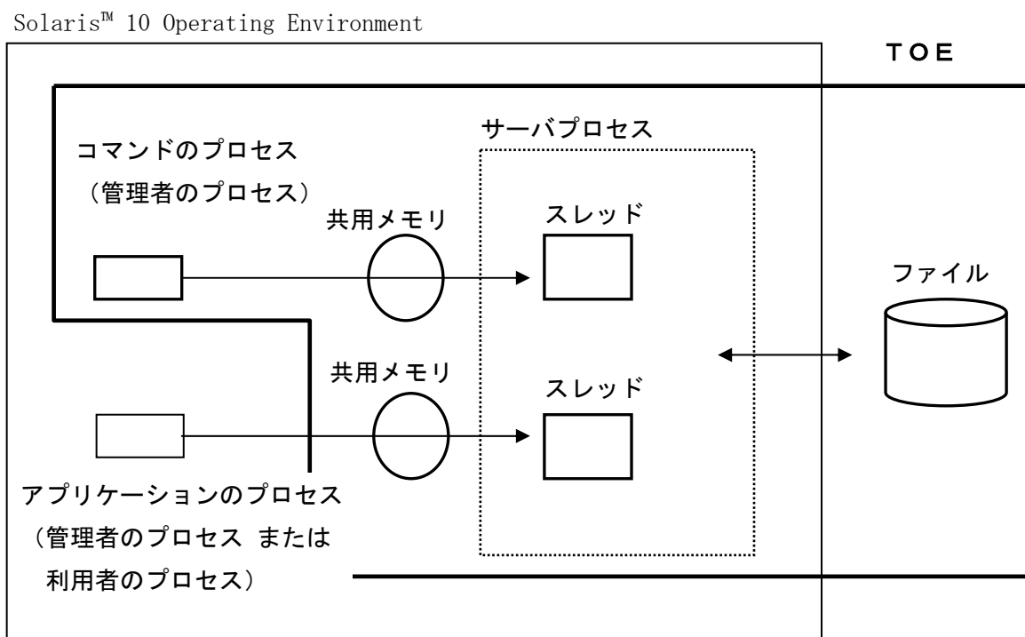
図2. 1 TOEのプロセス実行イメージ
