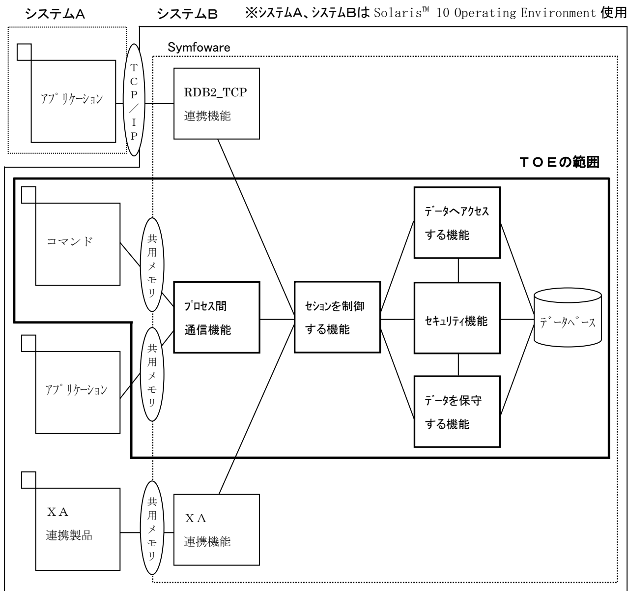
図 2. 2 機能構成
