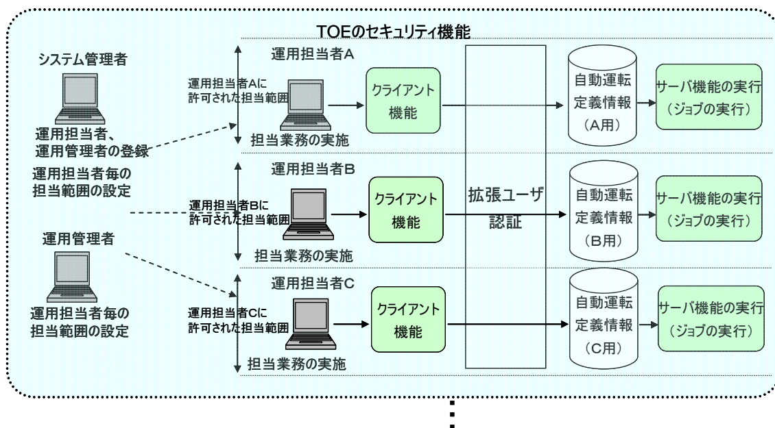
図 2-4 クライアント機能使用時のセキュリティ機能の動作イメージ
