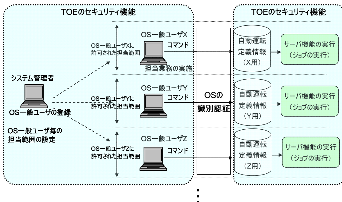
図 2-5 コマンド使用時のセキュリティ機能の動作イメージ
