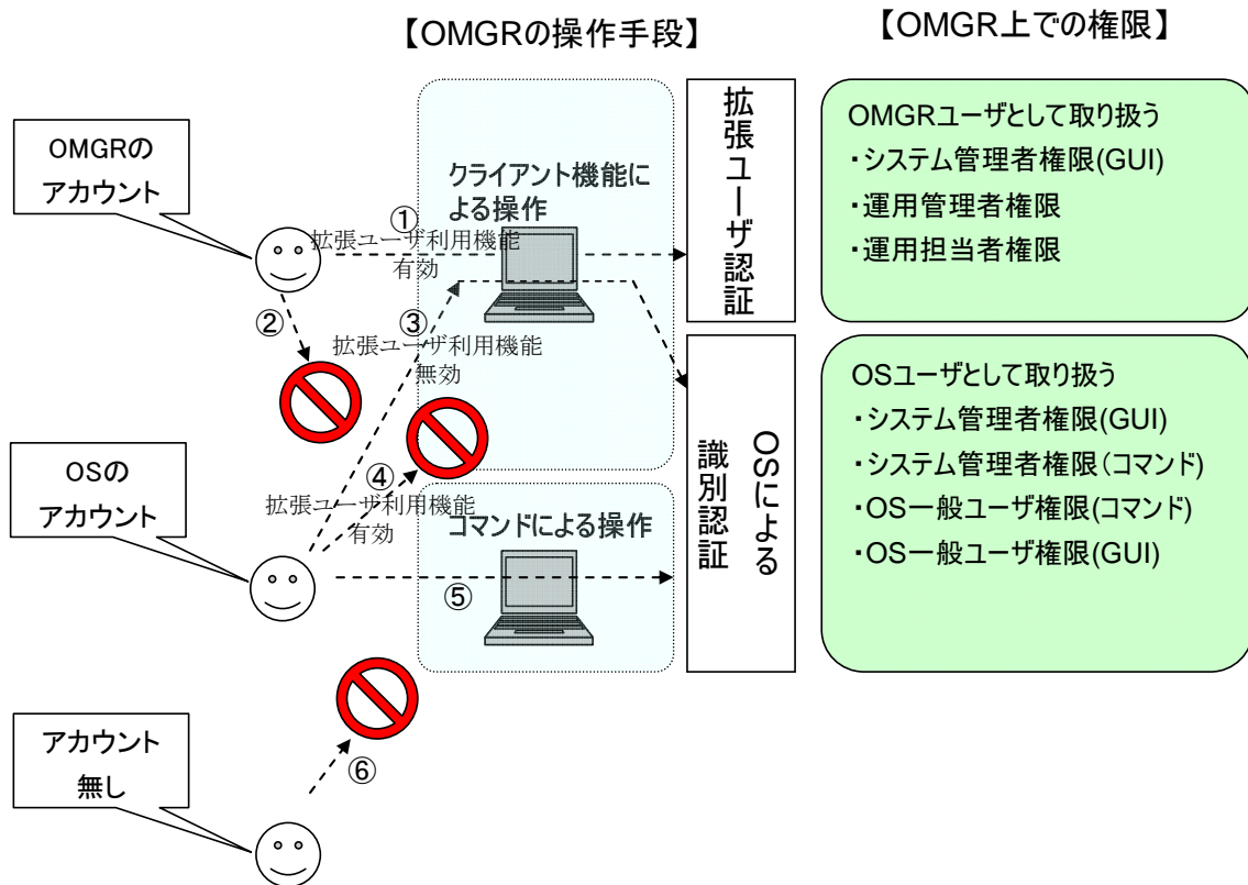
図 2-3 拡張ユーザ利用及び認証機能と関係者の関係イメージ
