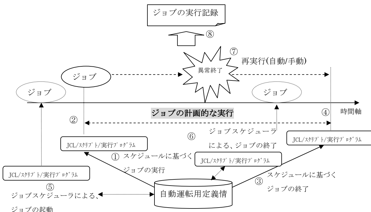
図 2-7 ジョブの計画的な実行
