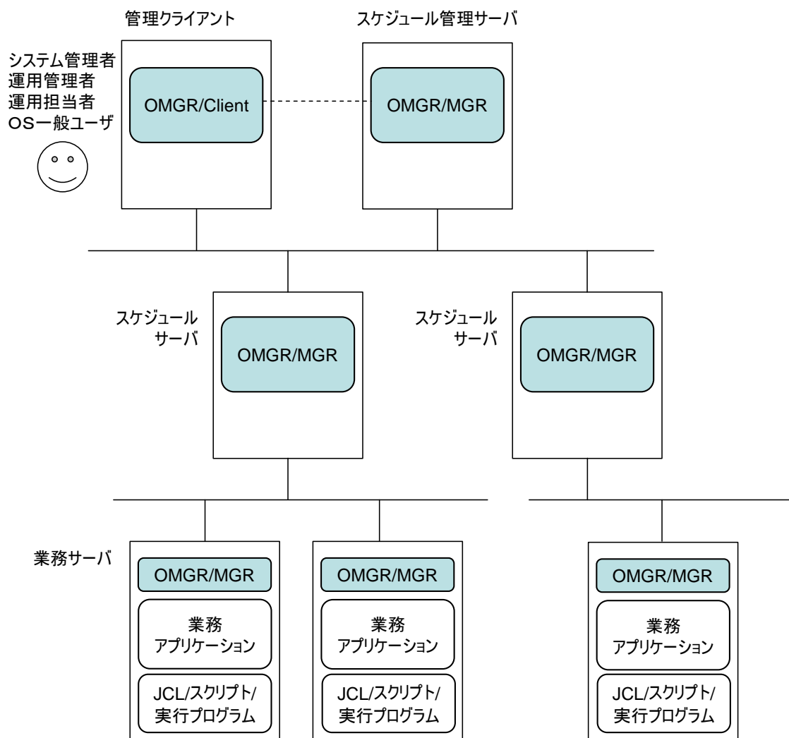
図 2-2 大規模システムにおける TOE の動作環境
