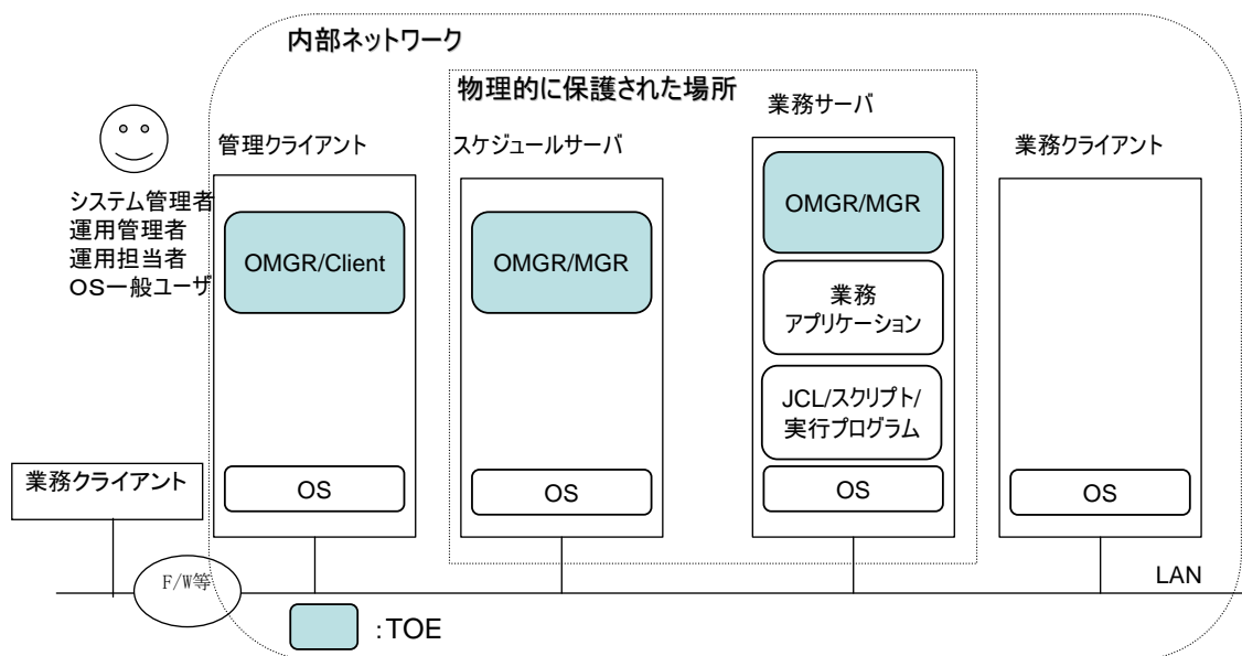
図 2-1 TOE の基本的な動作環境
