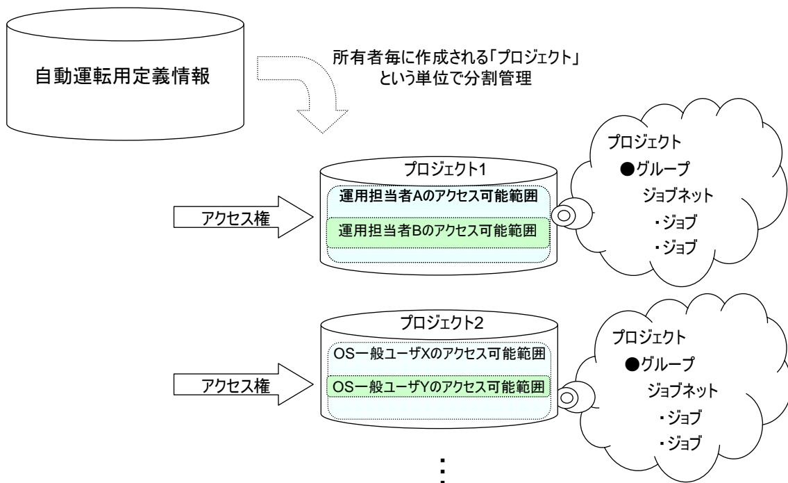
図 6-1 プロジェクト(自動運転用定義情報)とアクセス権の関係
