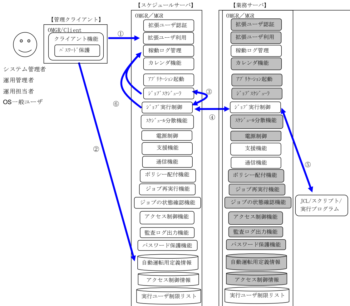
図 2-6 本 TOE の機能間の関係
