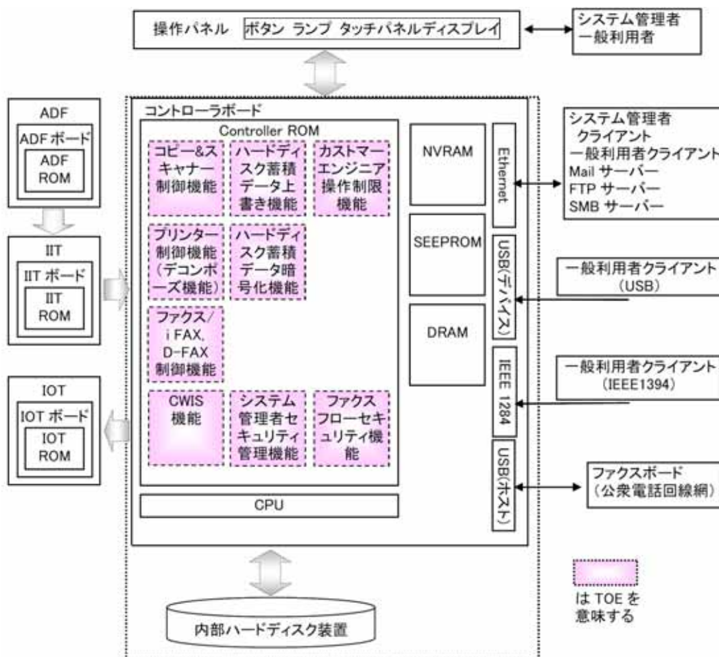
図1-1 TOEの物理的構成イメージ
