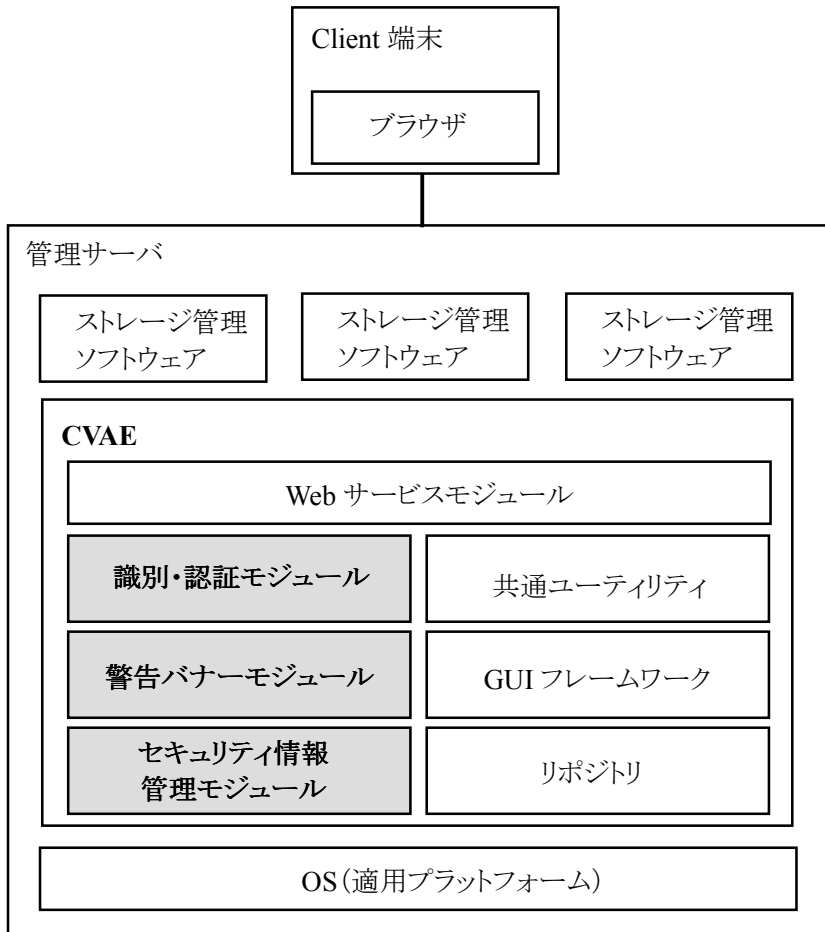
図 3 TOE を含めたソフトウェア構成図
