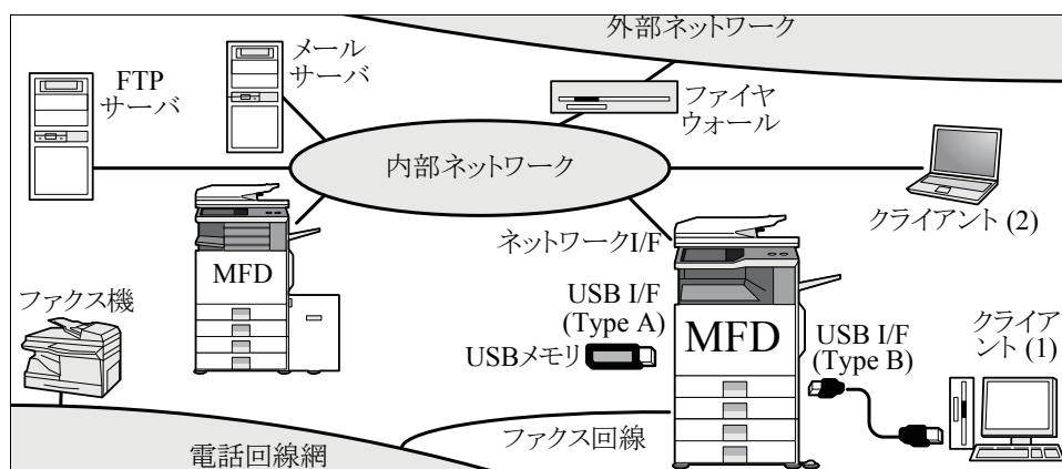
図 1: MFDの利用環境
