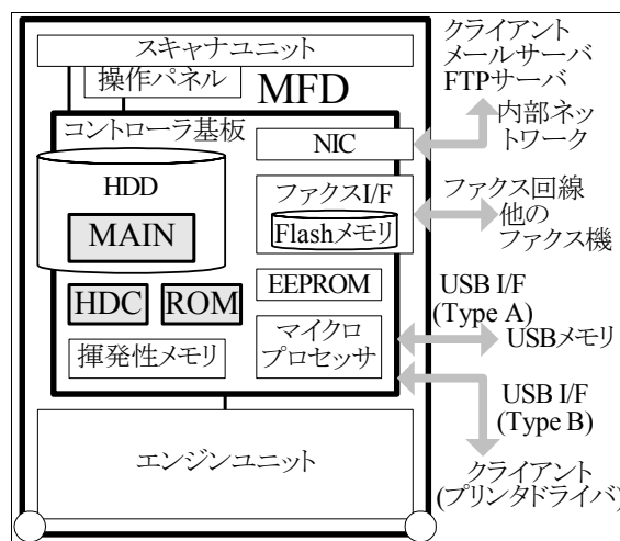
図 2: MFDの物理的構成とTOE
