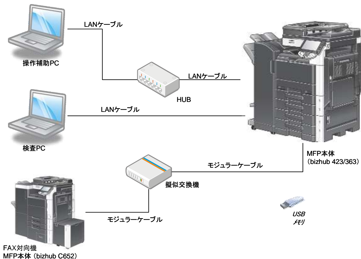
図7-2 侵入テストの構成図
