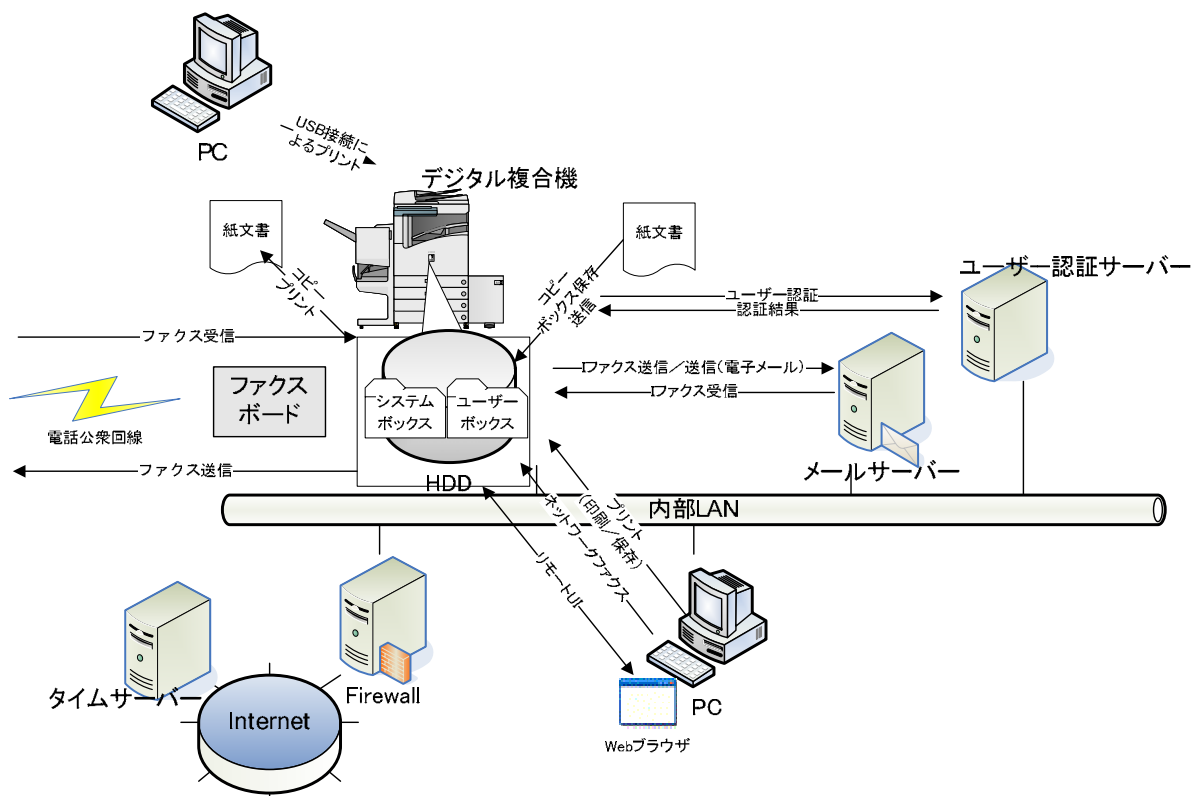
Figure 1 デジタル複合機の想定設置使用環境
