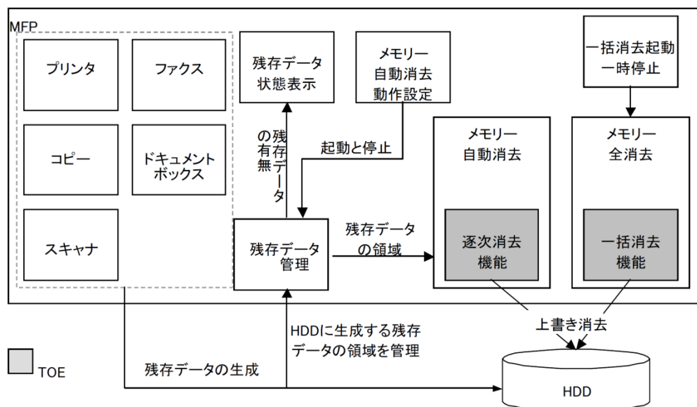
図5-1 TOEの構成と動作環境
