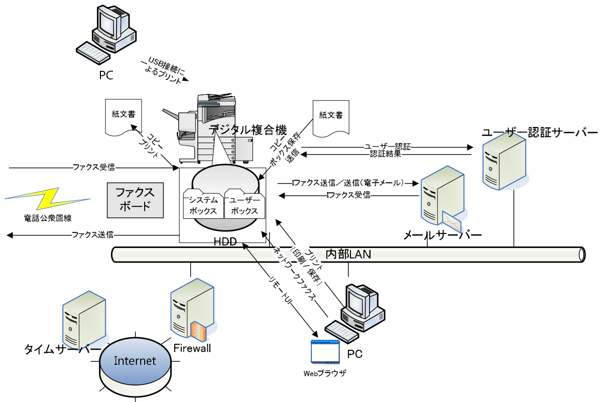
Figure 1 デジタル複合機< Canon imageRUNNER ADVANCE C5200 Series >の想定設置使用環境
