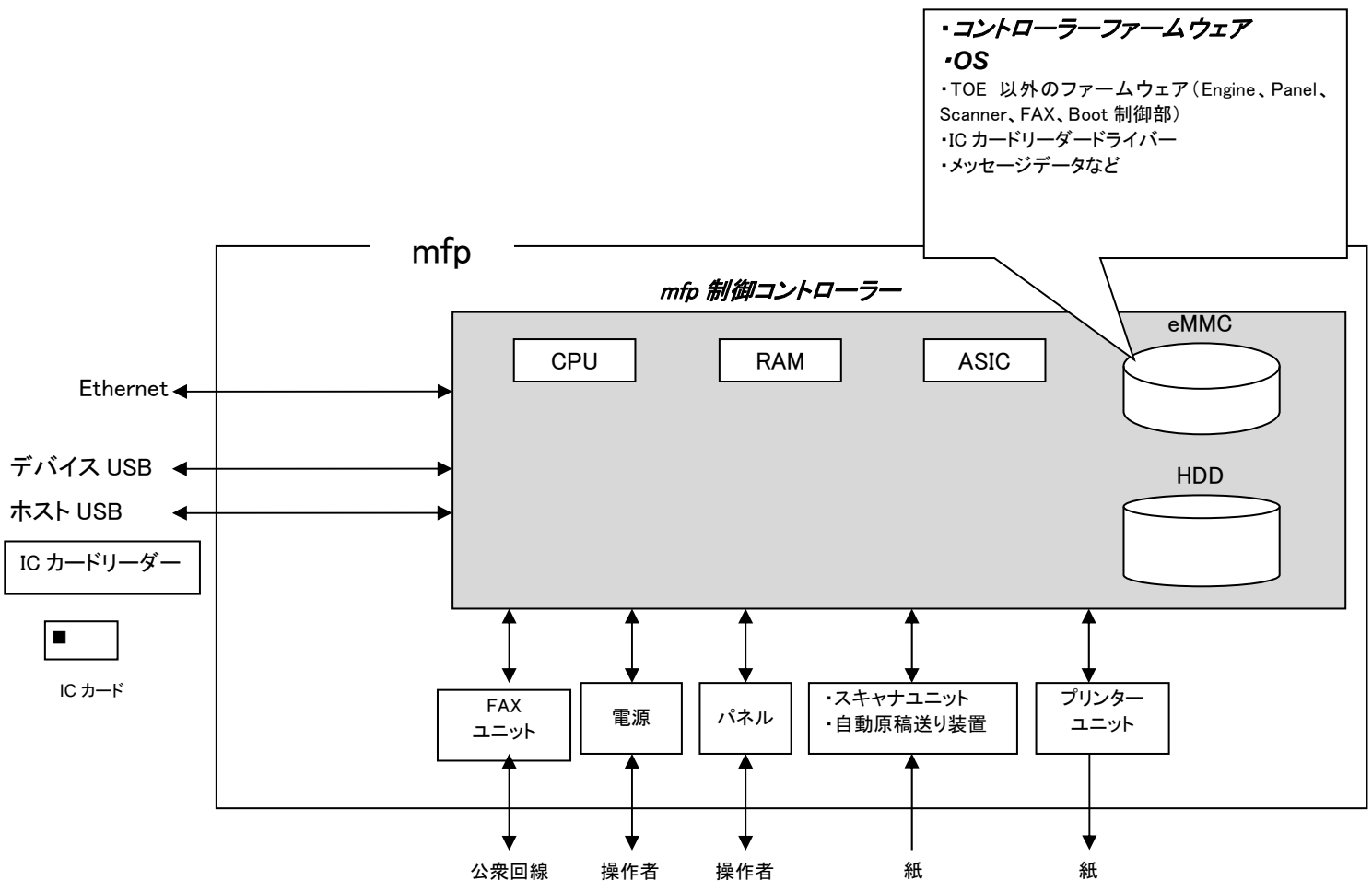
図 2 TOE に関するハードウェア構成
