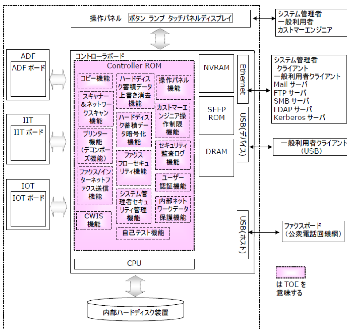
図 5-1 TOE境界
