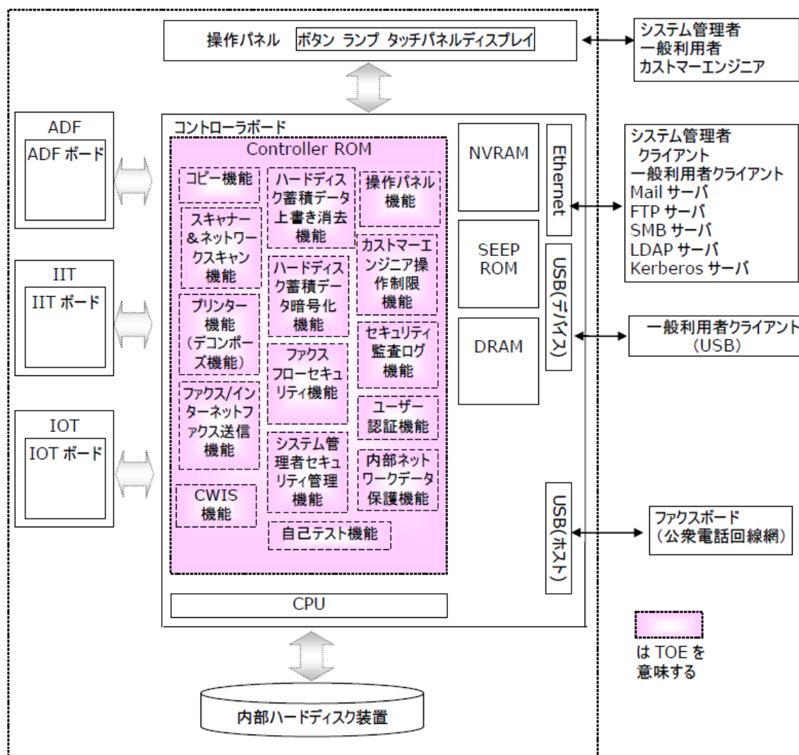
図 5-1 TOE境界
