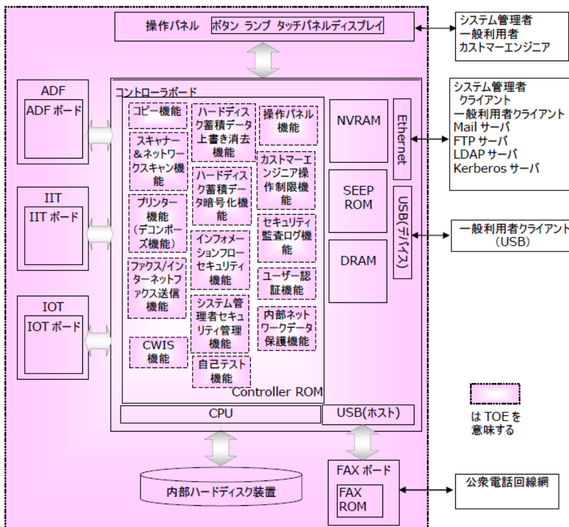
図 5-1 TOE の構成
