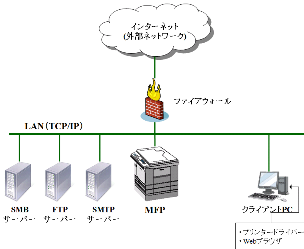
図 1：TOE の利用環境
