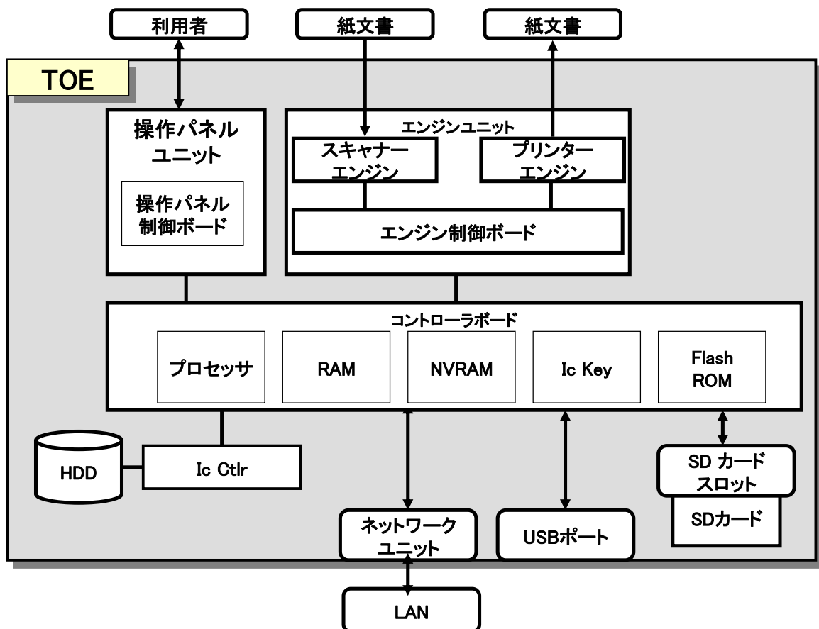
図 2：TOE のハードウェア構成
