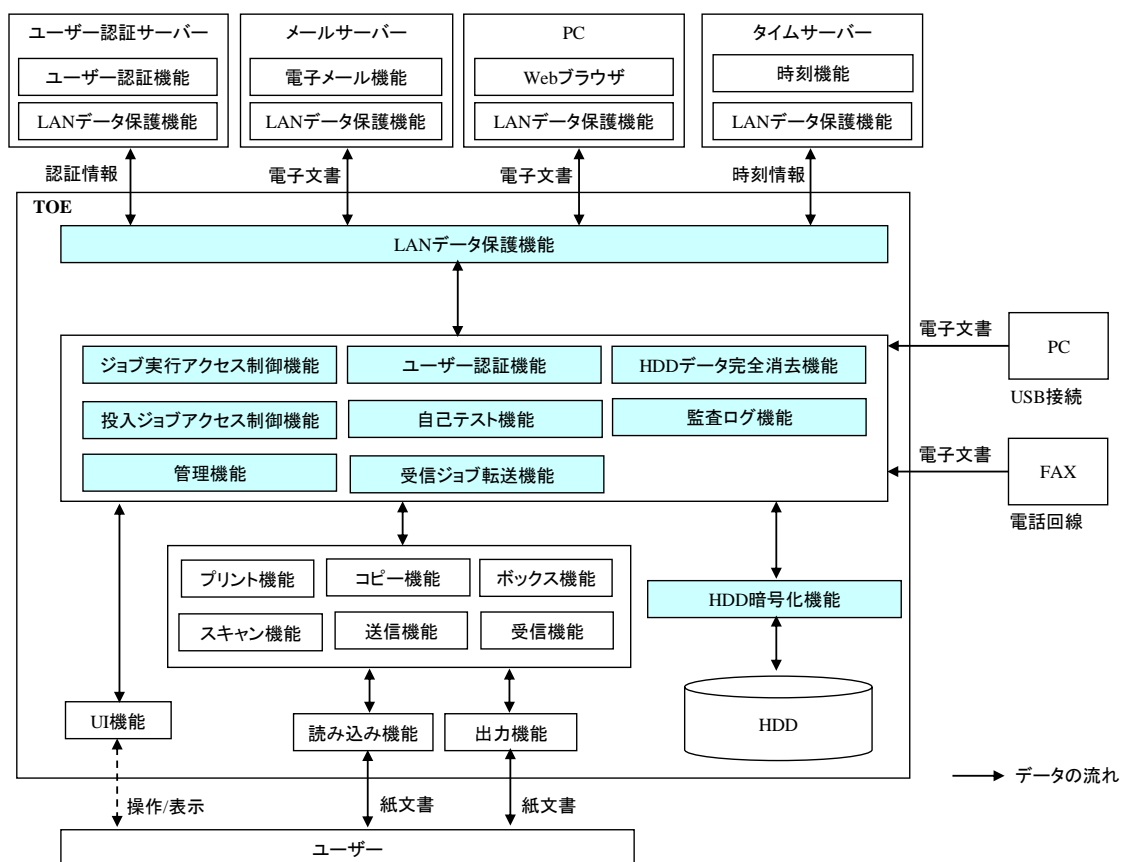
図5-1 TOE境界
