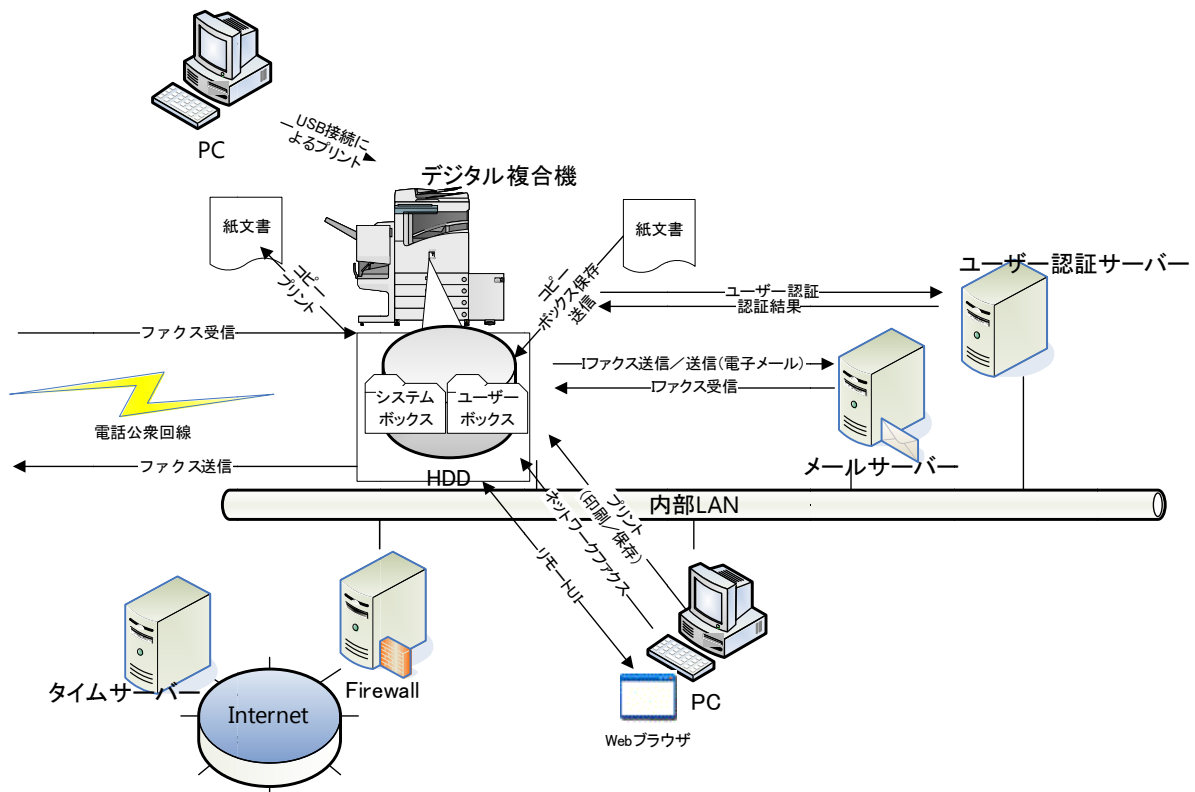
Figure 1 デジタル複合機< Canon imageRUNNER ADVANCE 8500 Series >の想定設置使用環境
