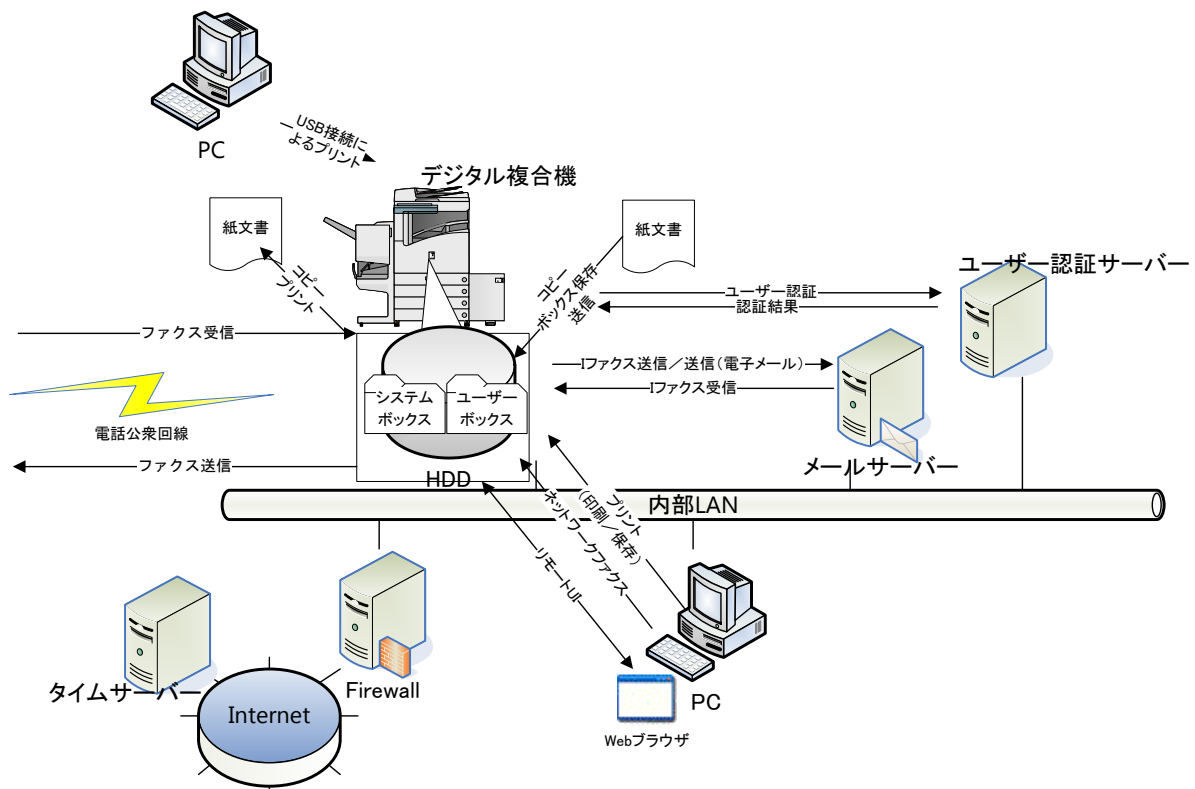
Figure 1 デジタル複合機< Canon imageRUNNER ADVANCE C35900KG/C3500 Series >の想定設置使用環境
