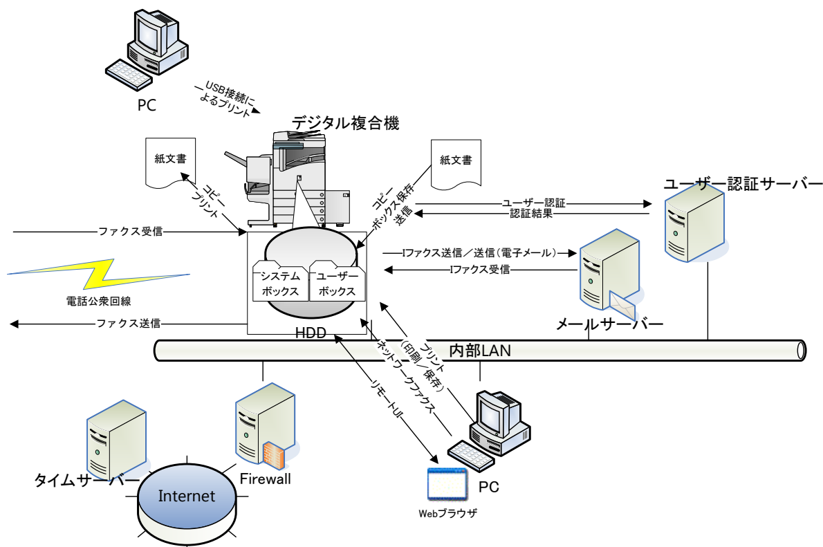
Figure 1 デジタル複合機< Canon imageRUNNER ADVANCE C75900KG/C7500 Series >の想定設置使用環境
