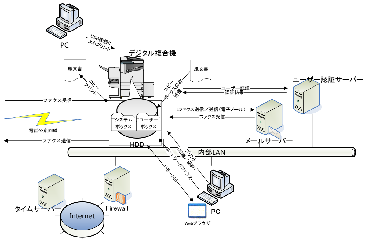
Figure 1 デジタル複合機< Canon imageRUNNER ADVANCE 6500 Series >の想定設置使用環境
