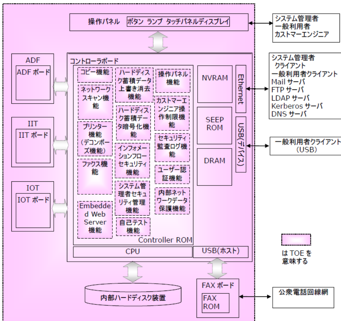
図 5-1 TOE の構成
