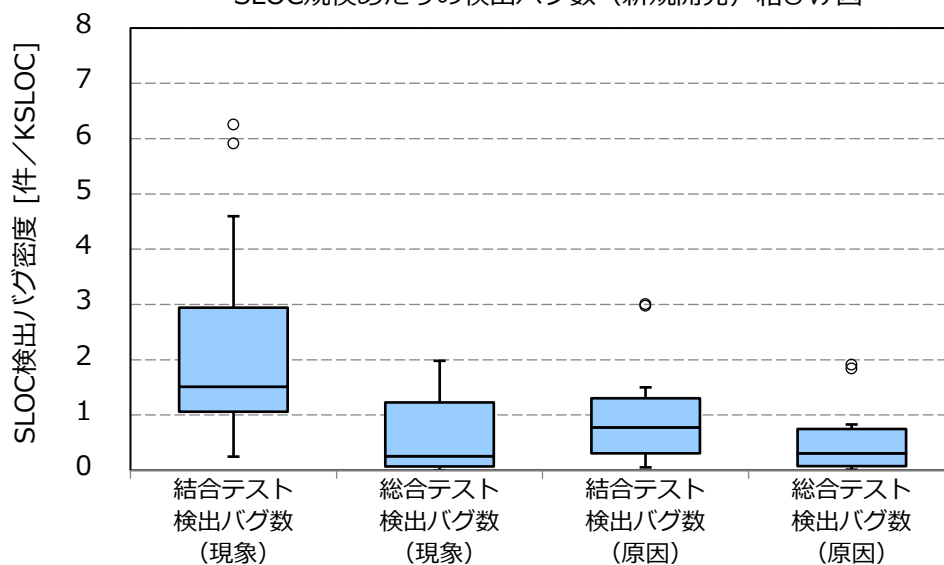
SLOC 規模あたりの検出バグ数 (新規開発) 箱ひげ図
