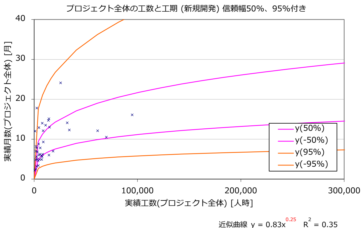
図 A3-3-1 プロジェクト全体の工数と工期(新規開発)(信頼区間 50%、95%付き)
