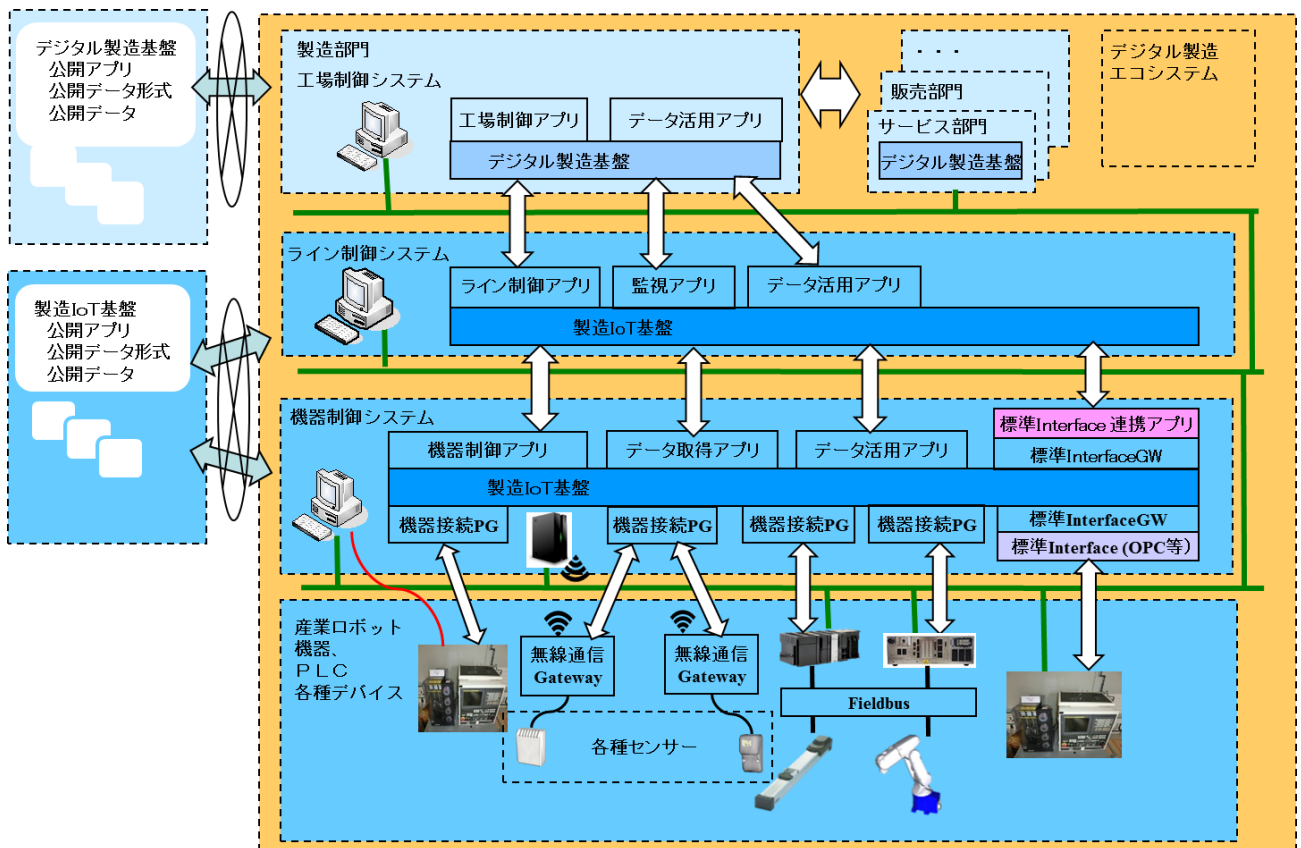
図 2.1-4 デジタル製造エコシステムの製造システムの概要
