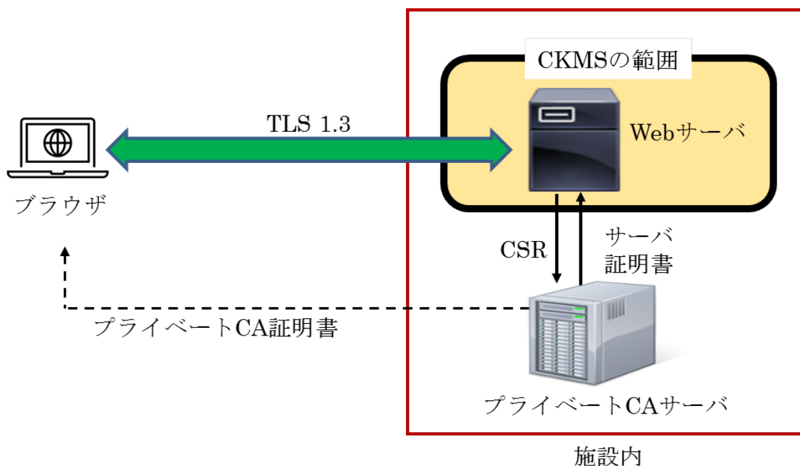
図 4-1 施設内 Web サーバシステム
