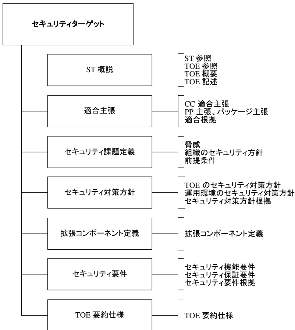
図 5 セキュリティターゲットの内容
