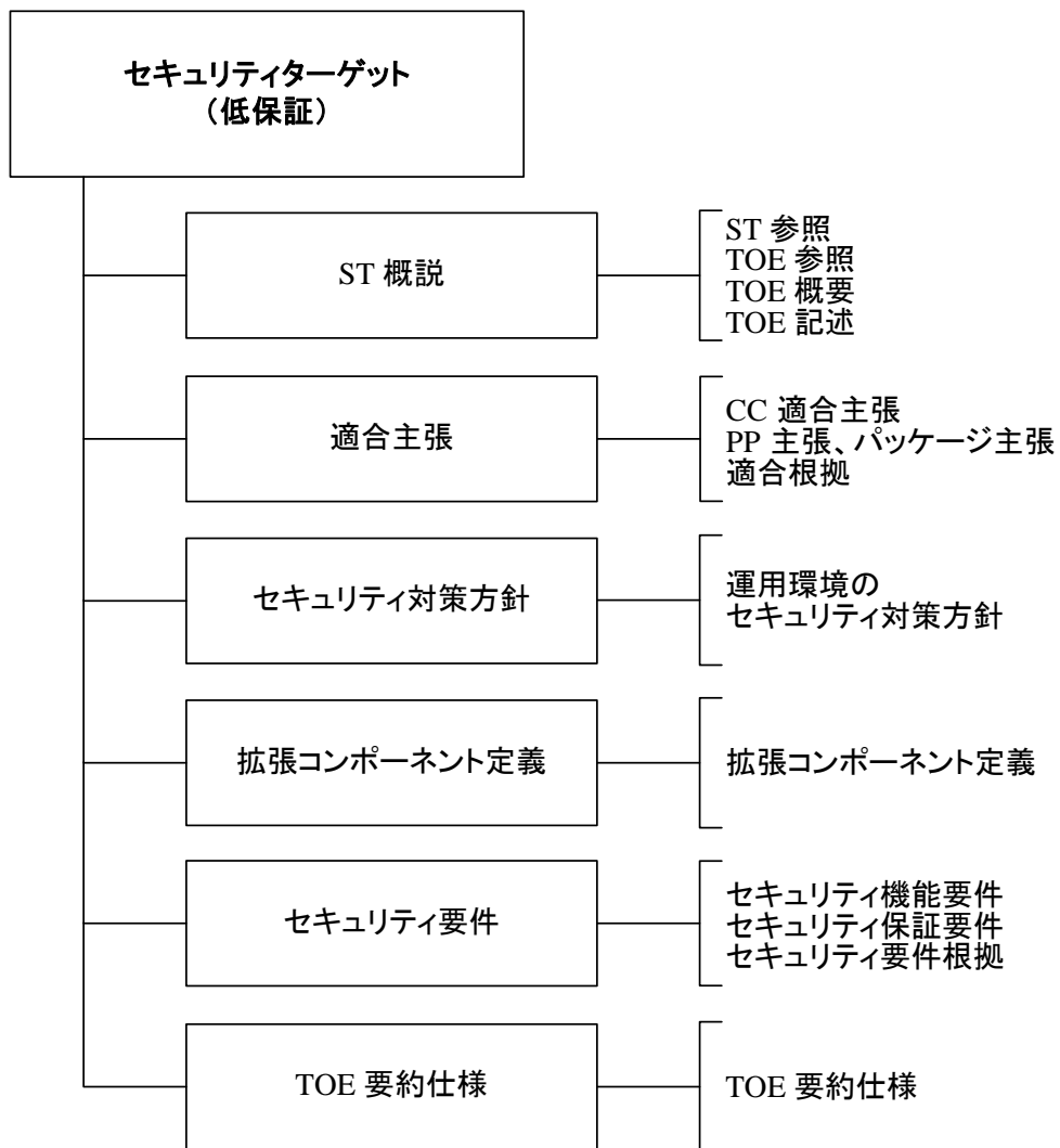
図 8 低保証セキュリティターゲットの内容
