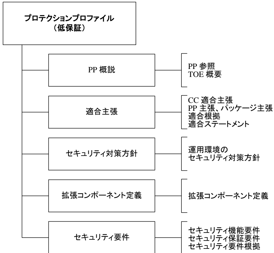
図 10 低保証プロテクションプロファイルの内容
