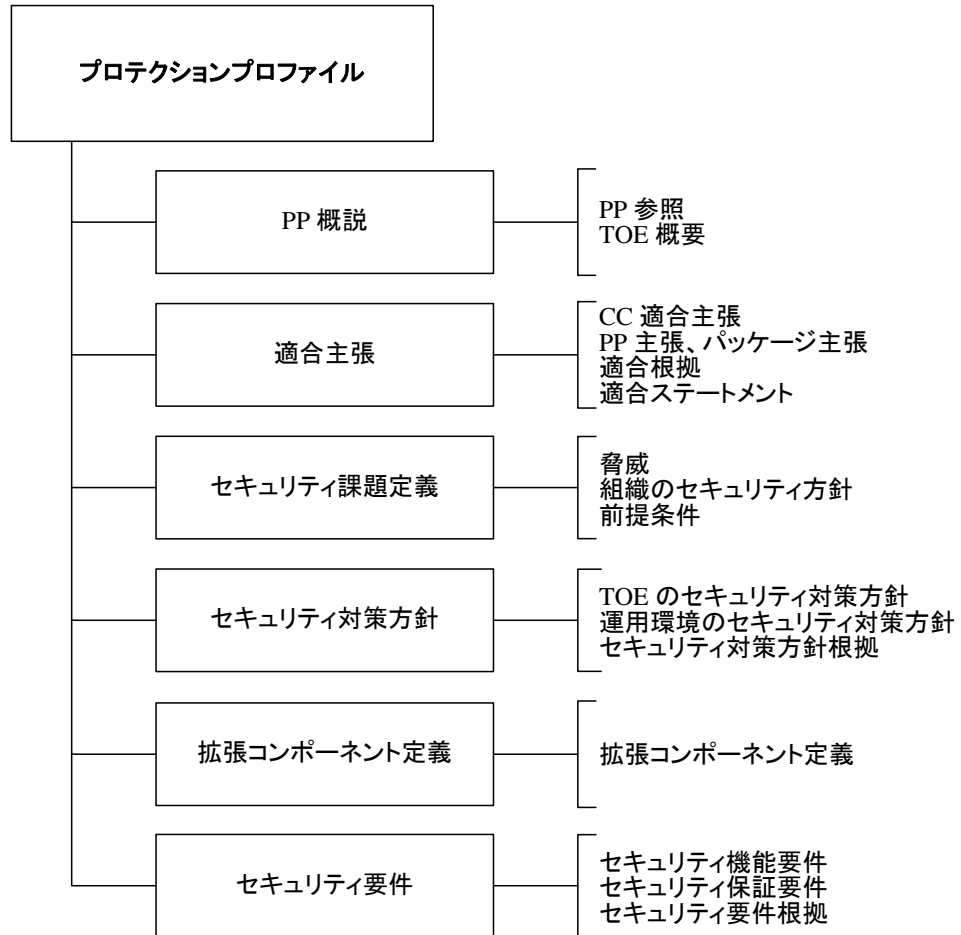
図 9 プロテクションプロファイルの内容
