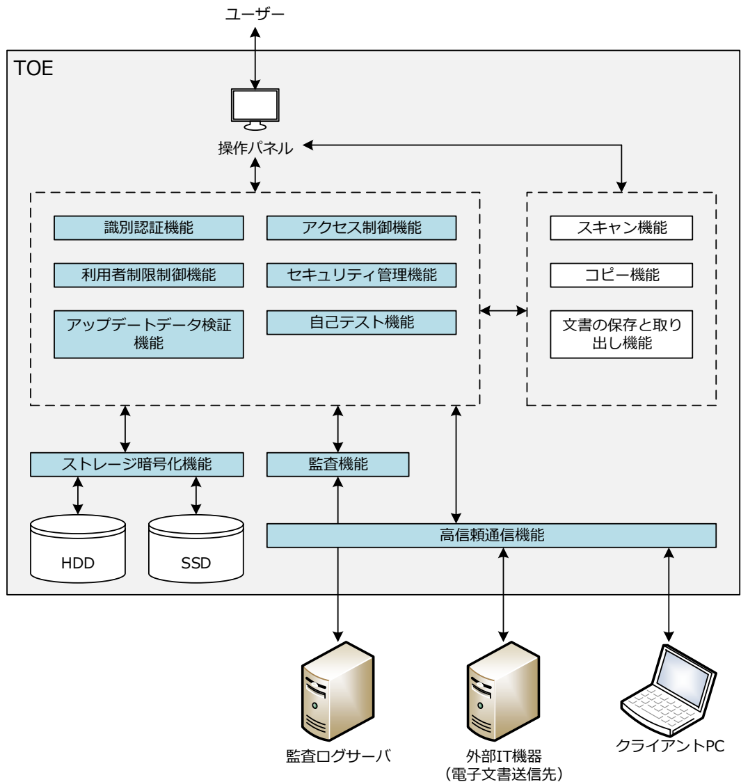
図 5-1 TOE の構成
