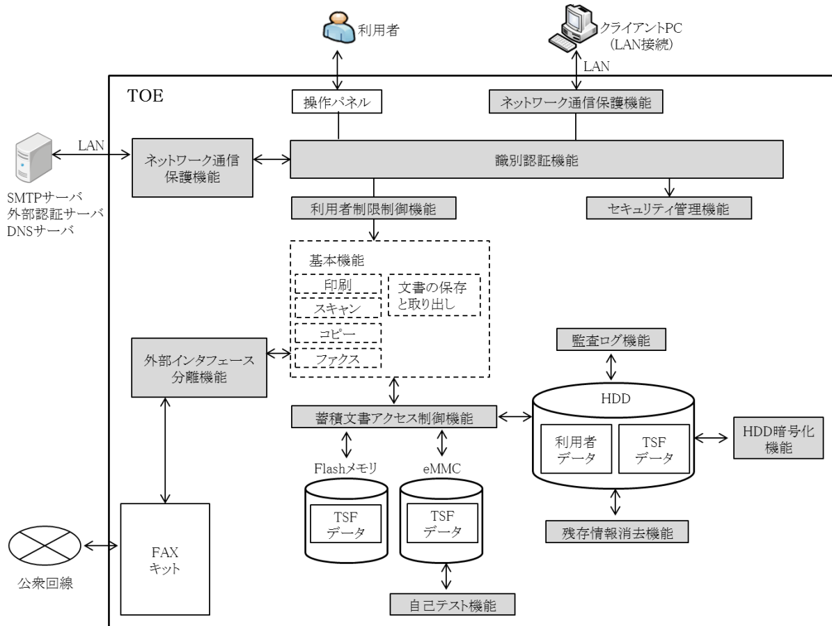
図5-1 TOEの構成
