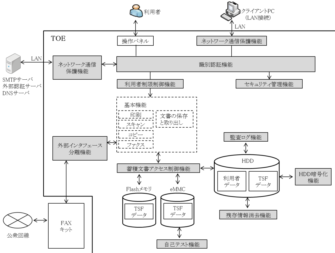
図5-1 TOEの構成
