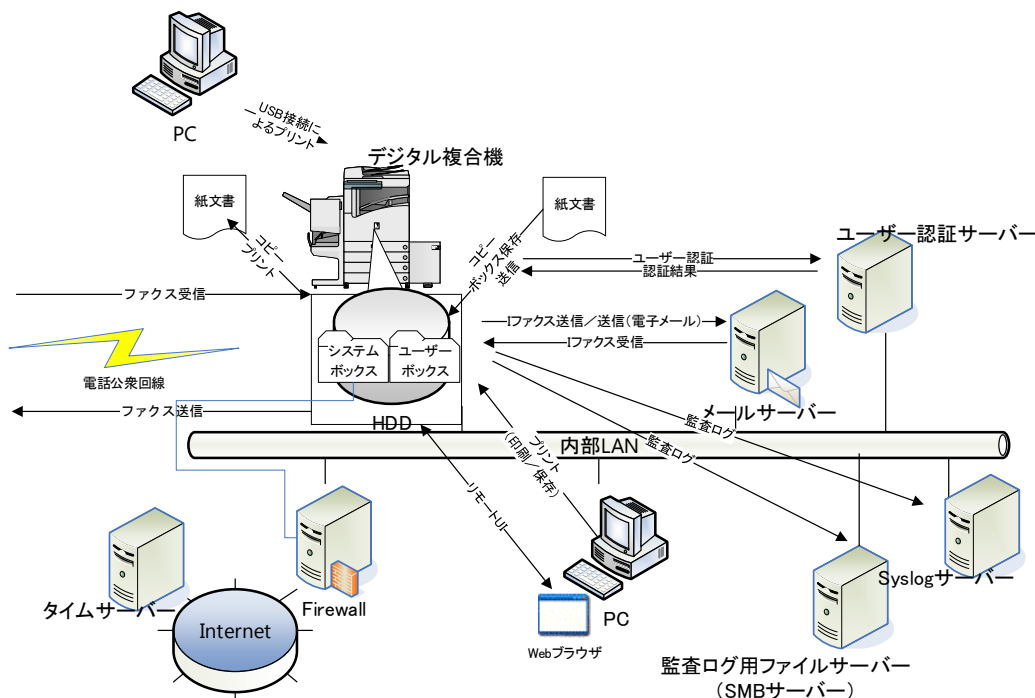
Figure 1 デジタル複合機< Canon imageRUNNER ADVANCE C35900KG (III)/ C3500 III Series ファクス付き>の想定設置使用環境
