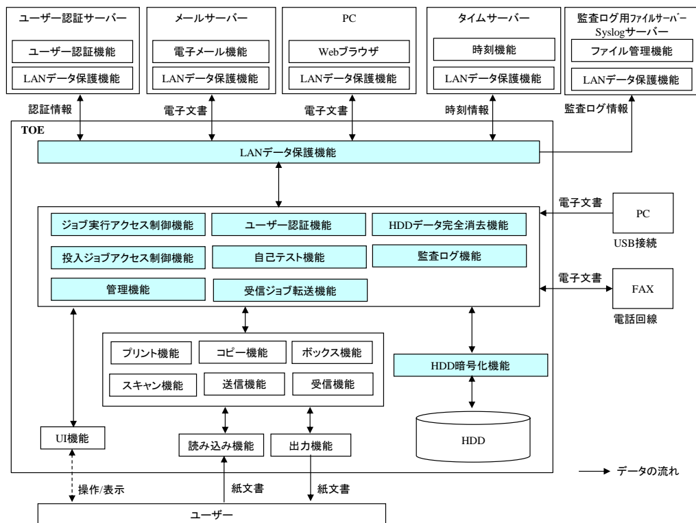
Figure 3 TOE の機能構成
