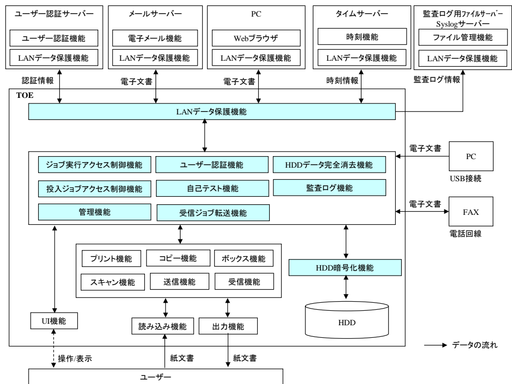
図 5-1 TOE 境界
