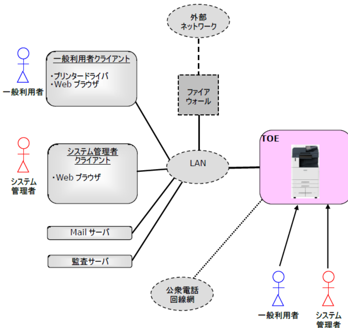
図4-1 TOEの運用環境（ファームウェア更新時を除く）
