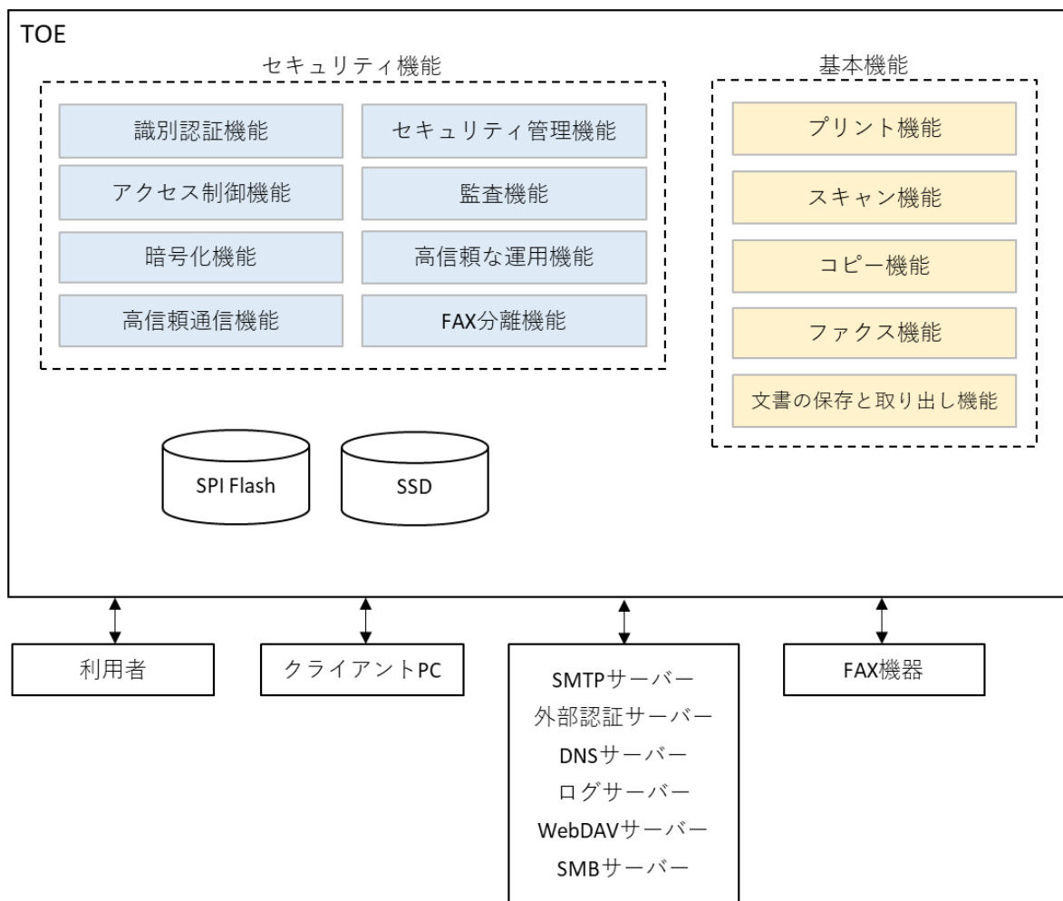
図 5-1 TOE の構成
