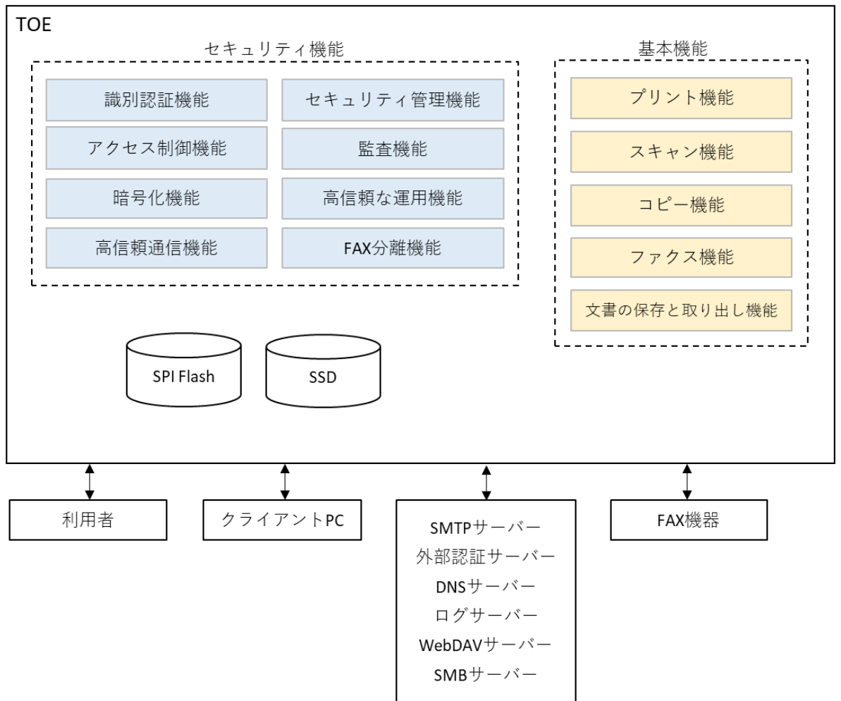
図 5-1 TOE の構成
