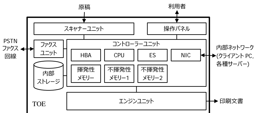
Figure 2: TOE の物理的構成
