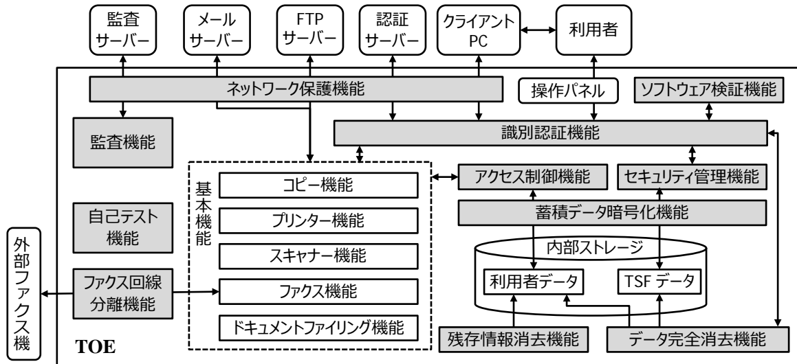
Figure 3: TOE の論理的構成
