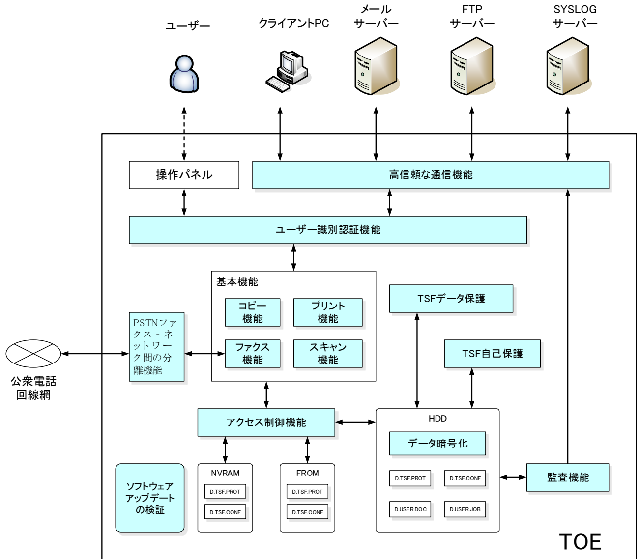
図5-1 TOE 境界
