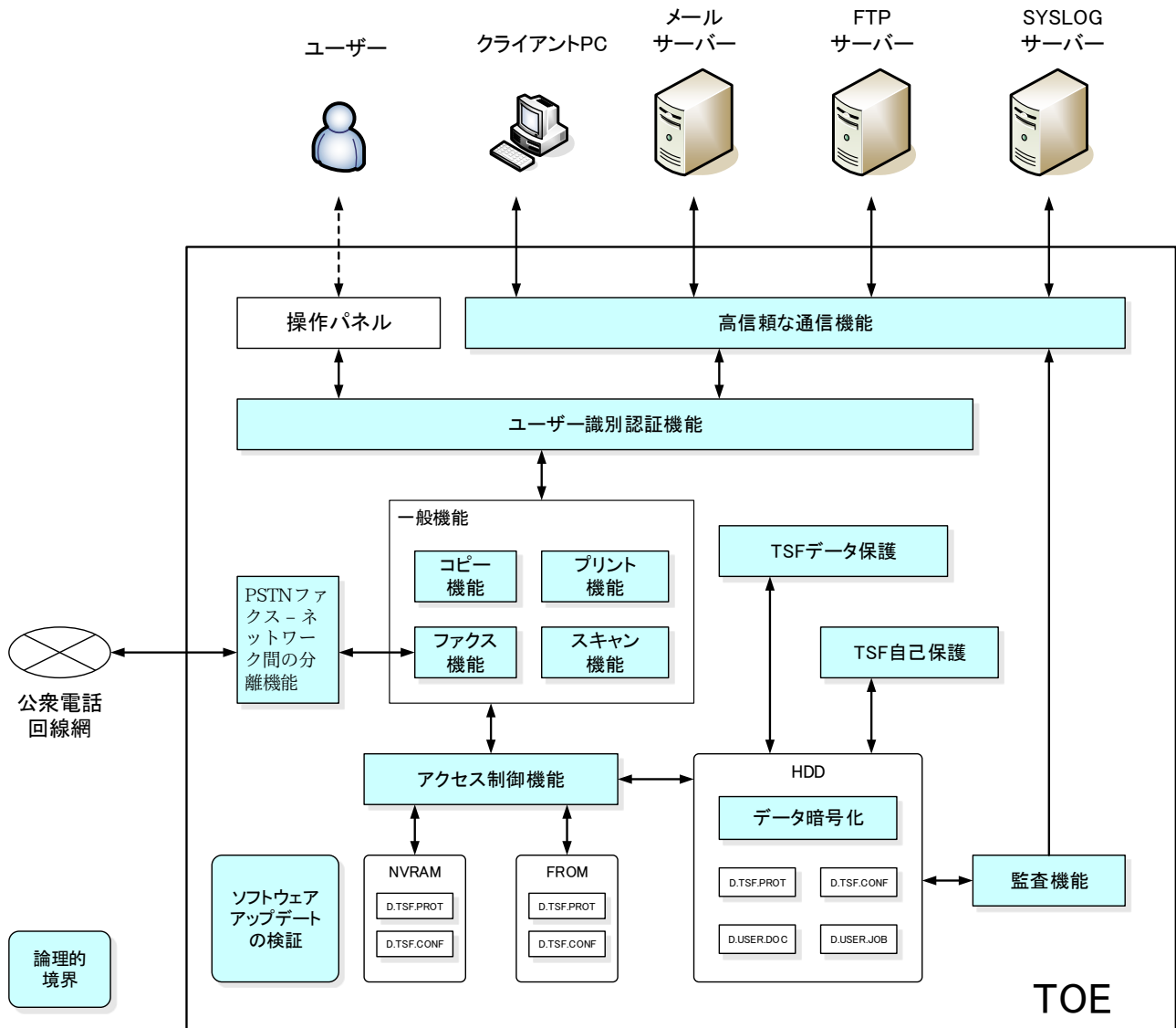
図3 論理的境界
