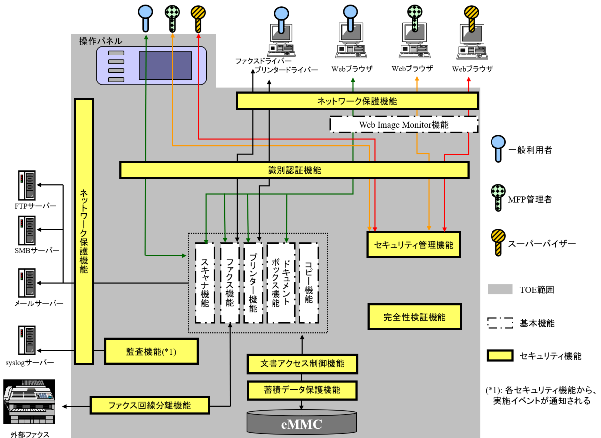
図5-1 TOEの構成
