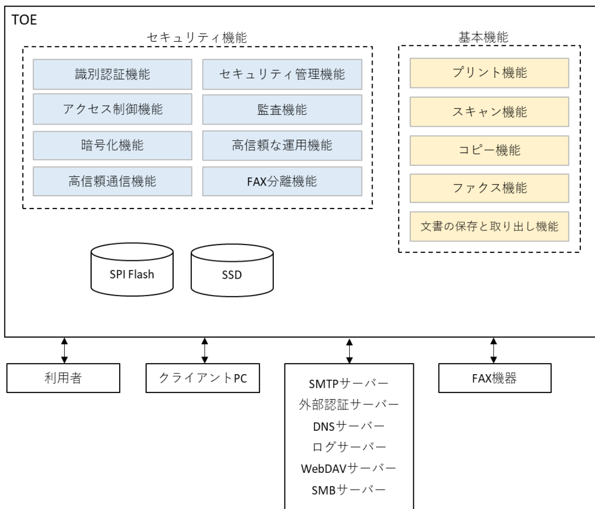
図 5-1 TOE の構成
