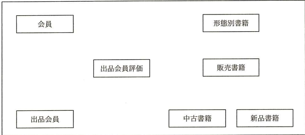
図1 B君が設計した概念データモデル（未完成）
