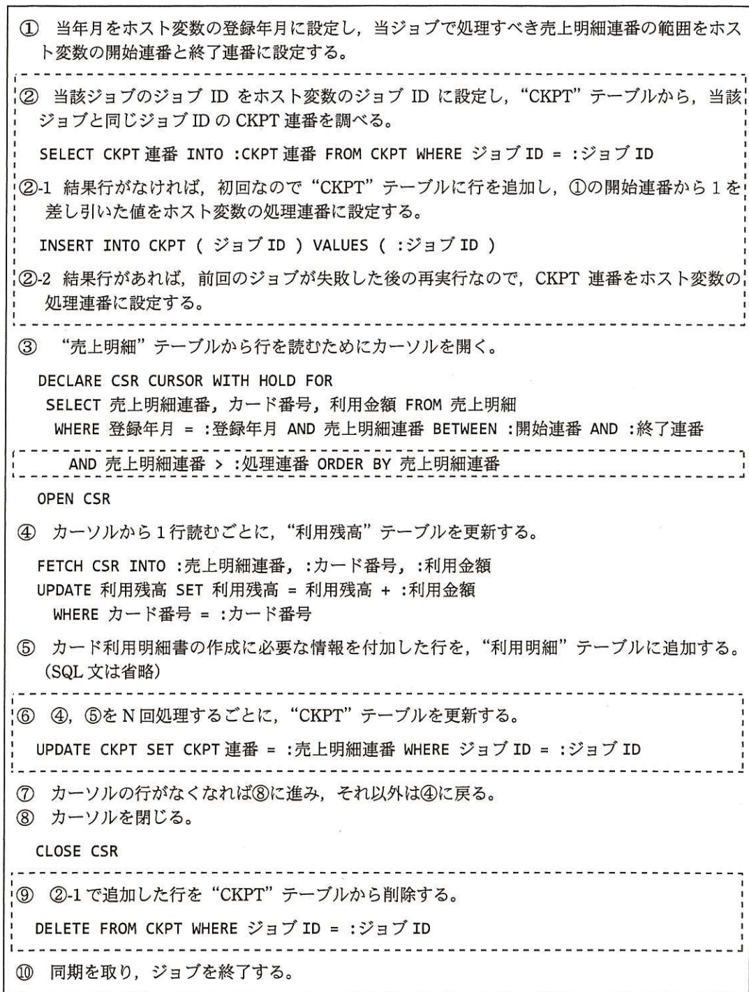
図 3 C/R 機能を追加した後のプログラムの処理の流れと SQL 文（一部省略）
