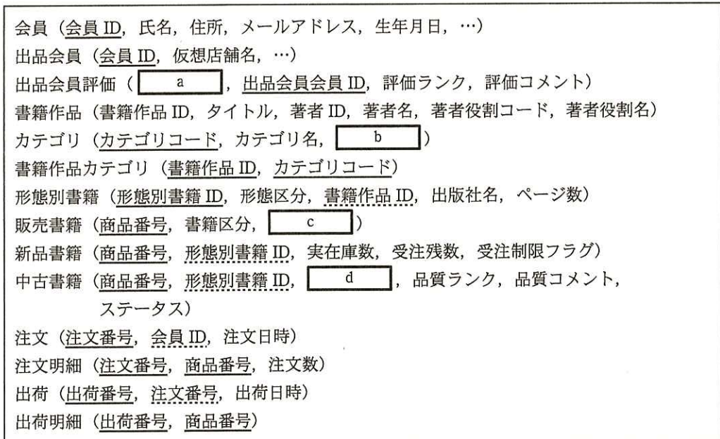
図2 B君が設計した関係スキーマ（未完成）
